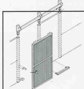
A - Porte coulissante
