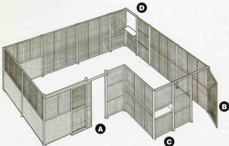
A - Porte coulissante
